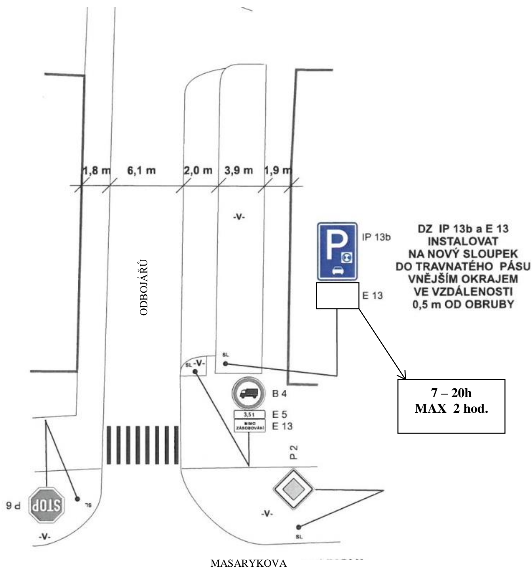
Obr. 1: Situace dopravního značení – ulice Odbojářů
