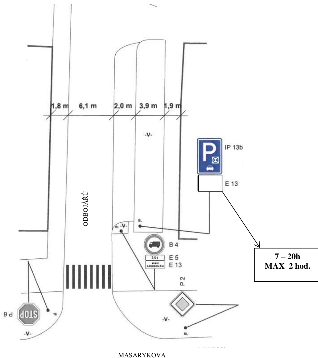
Obr. 1: Situace dopravního značení – ulice Odbojářů
